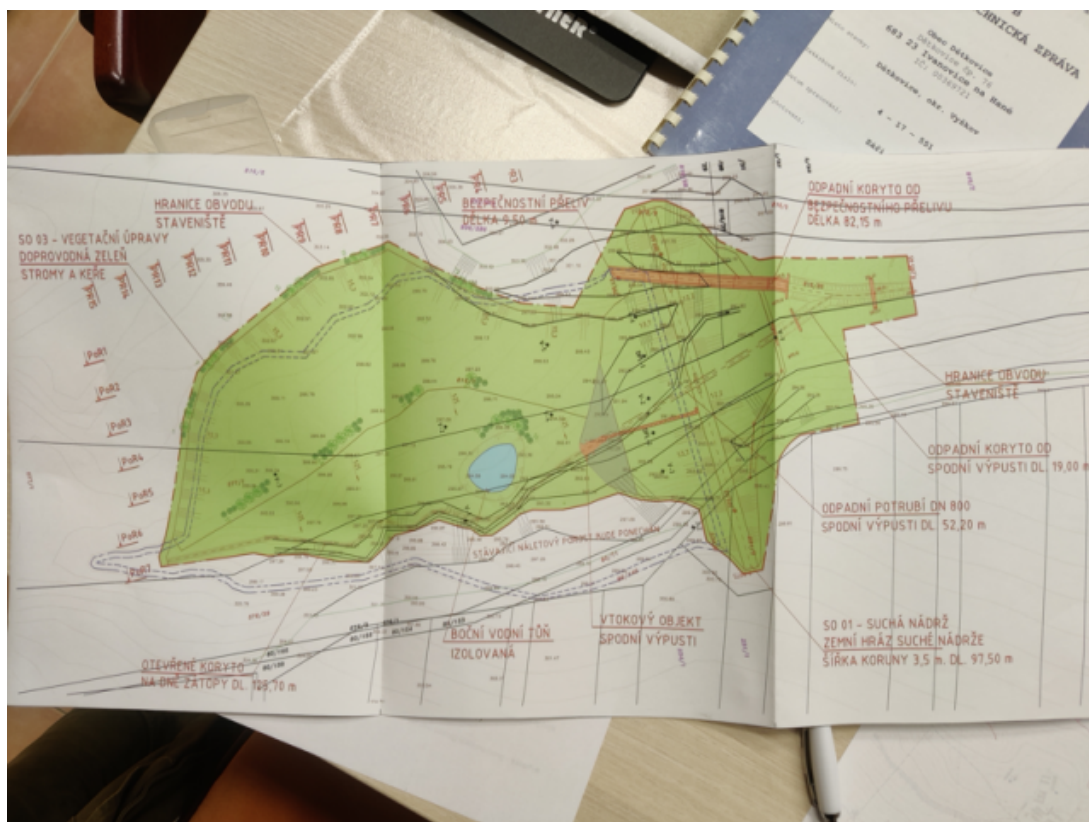
Obr. 6: Situační výkres suchého poldru Dětkovice
